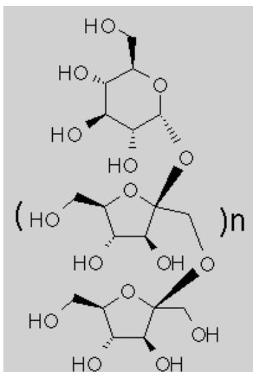
Figura 1. Molécula de inulina
