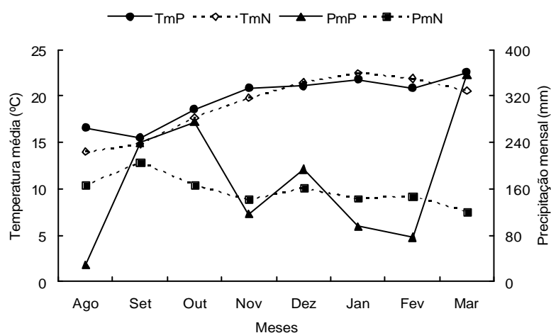
Figura 1. Precipitação mensal (PmP) e temperatura média mensal (TmP) durante o período experimental e as normas para a região (Precipitação mensal normal, PmN; temperatura média mensal normal, TmN). Passo Fundo, Rio Grande do Sul, Brasil, 2001/2002. Fonte: Embrapa Trigo ( www.cnpt.embrapa.br ).
