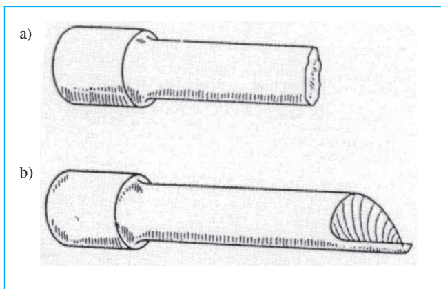
Fig. 3. Tipos de falla en probetas sometidas a tracción.
