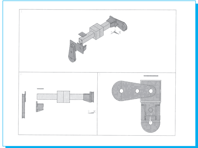
Fig. 5. Soporte de reductor trasero para tractor.
