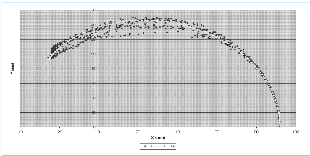
Fig. 15. Trayectoria descrita por las funciones descriptivas del dedo Índice en el agarre cilíndrico.
