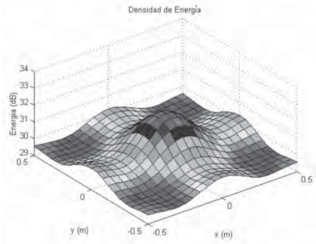
Figura 10. Distribución de la densidad de energía aproximada, obtenida con el método de Galerkin, en una placa de aluminio simplemente apoyada cuando \eta=0.10 y f=487 Hz.
