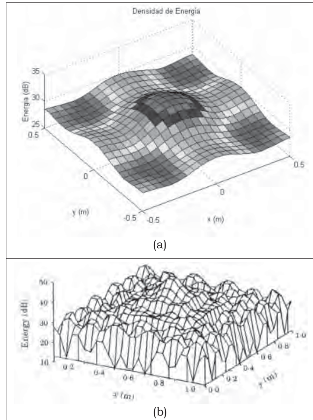
Figura 7. Distribución de la densidad de energía en una placa de aluminio simplemente apoyada, con \eta=0.20 y f=239 Hz, obtenida con (a) la solución aproximada con el método de Galerkin y (b) la solución exacta reportada por Bouthier y Bernhard (1993).
