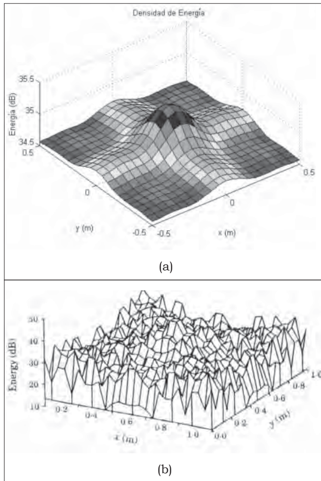
Figura 9. Distribución de la densidad de energía en una placa de aluminio simplemente apoyada, con \eta=0.05 y f=487 Hz, obtenida con (a) la solución aproximada con el método de Galerkin y (b) la solución exacta reportada por Bouthier y Bernhard (1993).
