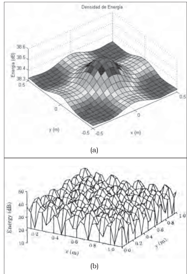
Figura 5. Distribución de la densidad de energía en una placa de aluminio simplemente apoyada, con \eta=0.05 y f=239 Hz, obtenida con (a) la solución aproximada con el método de Galerkin y (b) la solución exacta reportada por Bouthier y Bernhard (1993).
