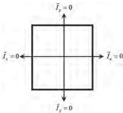
Figura 2. Condiciones de frontera, intensidad de energía nula en los extremos, para la placa de aluminio simplemente apoyada.
