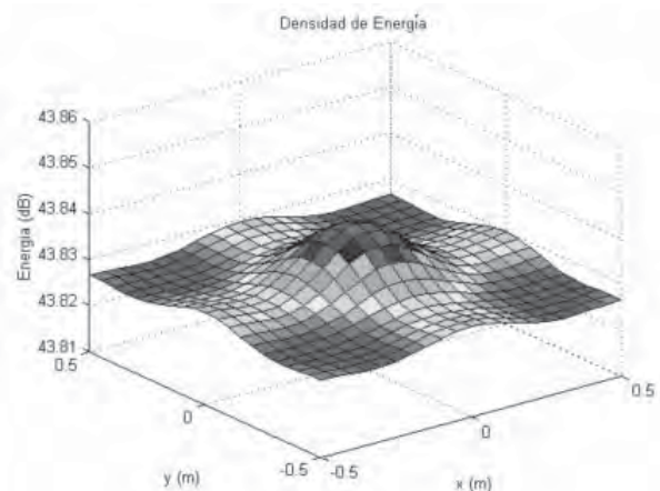
Figura 8. Distribución de la densidad de energía aproximada, obtenida con el método de Galerkin, en una placa de aluminio simplemente apoyada cuando \eta=0.01 y f=487 Hz.
