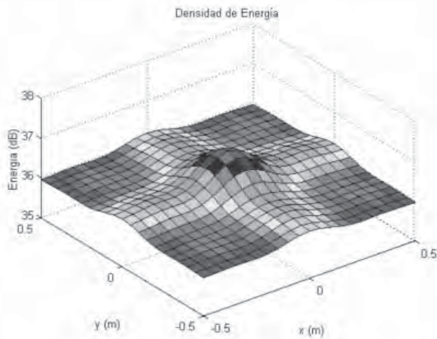
Figura 6. Distribución de la densidad de energía aproximada, obtenida con el método de Galerkin, en una placa de aluminio simplemente apoyada con \eta=0.10 y f=239 Hz.
