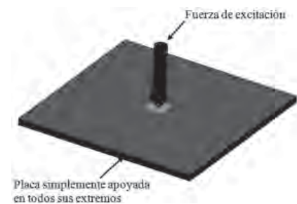
Figura 3. Placa cuadrada simplemente soportada de aluminio sujeta a una fuerza de excitación armónica, la cual actúa sobre un área de 0.1 \times 0.1 \text{ m}^2 en el centro de la placa.
