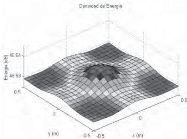
Figura 4. Distribución de la densidad de energía aproximada, obtenida con el método de Galerkin, en una placa de aluminio simplemente apoyada con \eta=0.01 y f=239 Hz.
