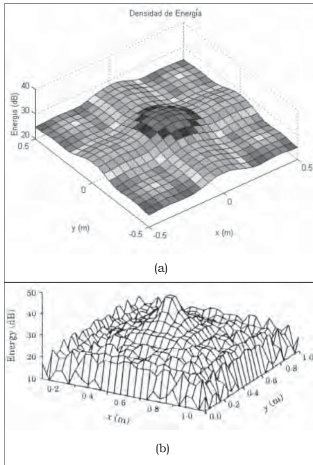
Figura 11. Distribución de la densidad de energía en una placa de aluminio simplemente apoyada, con \eta=0.20 y f=487 Hz, obtenida con (a) la solución aproximada con el método de Galerkin y (b) la solución exacta reportada por Bouthier y Bernhard (1993).
