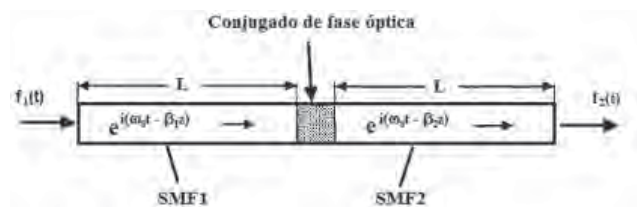
Figura 2. Diagrama esquemático de un compensador de dispersión cromática en una fibra óptica por medio del uso del conjugado de fase óptica.
