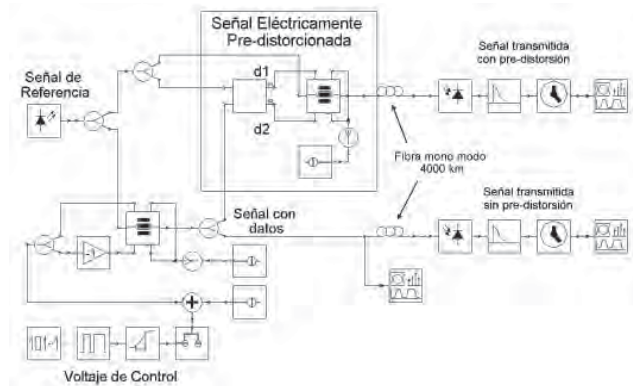
Figura 8. Diagrama de las simulaciones realizadas para la implementación del pre-compensador electrónico en el transmisor.
