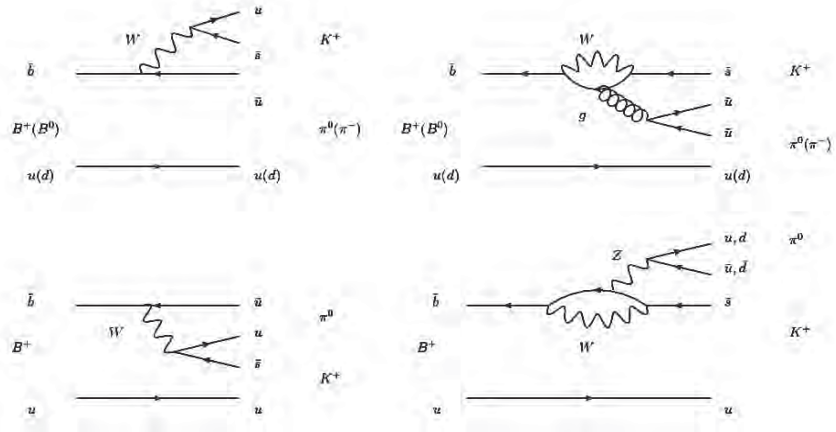
Figura 1. Diagramas de Feynman contribuyendo a los procesos bajo estudio.
