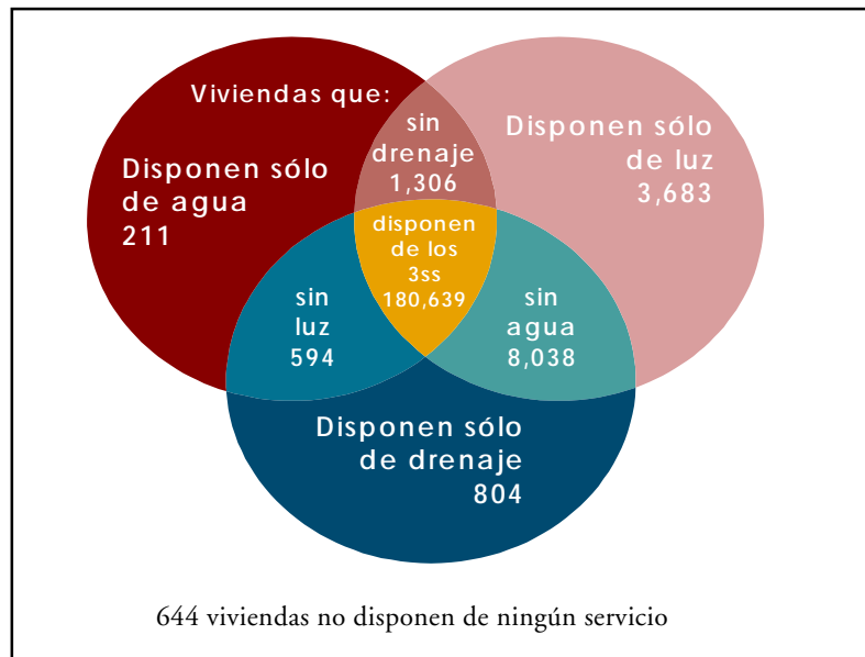
Figura 1. Aplicación del teorema inclusión-exclusión.
