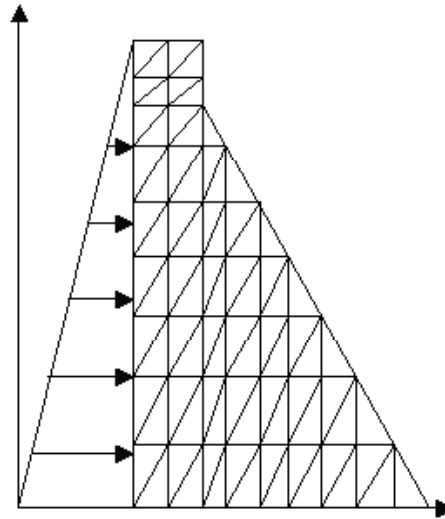
Figura 1. Discretización de una presa en Elementos Finitos. Cargas externas que modelan la presión hidrostática en la presa.
