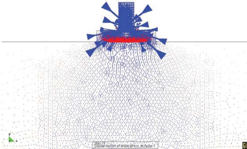
Figura 12. Distribución de esfuerzos principales en Zapata Corrida.
