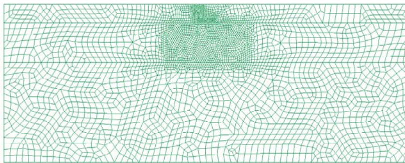
Figura 15. Malla de 3800 elementos cuadriláteros de 8 nodos (11617 nodos).
