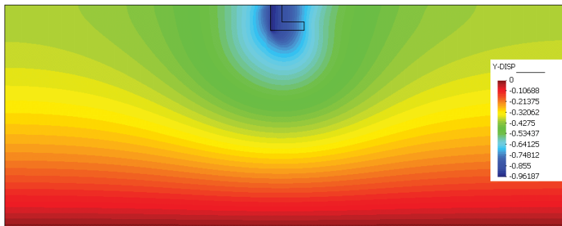
Figura 16. Desplazamientos verticales en Zapata Corrida de Colindancia.
