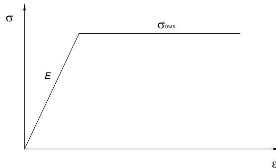
Figura 5. Ley constitutiva para material elastoplástico perfecto.
