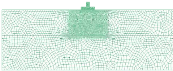
Figura 9. Malla de 4680 elementos cuadriláteros de 8 nodos (14309 nodos).
