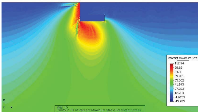
Figura 20. Razón entre esfuerzo máximo actuante y resistente en Zapata Corrida de Colindancia.
