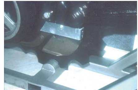
Lámina 93 Detalle de abridor de surco de ranura transversal (T. Friedrich)
