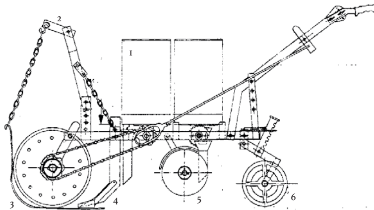
Figura 16 Diseño básico de una plantadora directa de tracción animal (Adaptado de Riveira y otros.)
