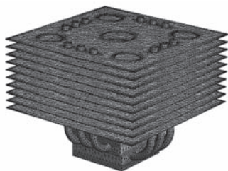
Figura 14. Malla de elementos finitos utilizada en la discretización del disipador de calor.
