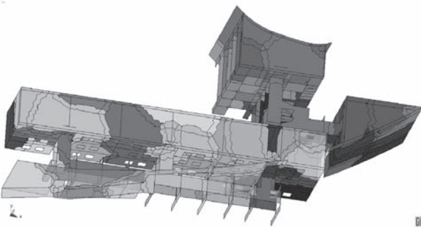
Figura 9. Descomposición de dominios del edificio.
