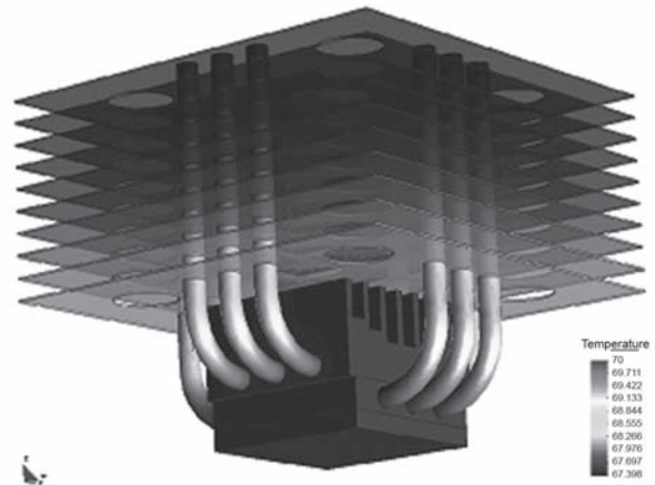
Figura 15. Isocontornos de temperatura en el Disipador.
