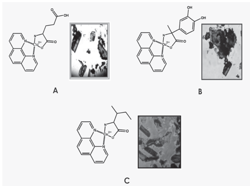
Figura 1. Estructura química y forma cristalina de los complejos de coordinación de [Cu(1,10-fenantrolina)(\text{aminoácidos})]^+ . En A) Complejo AG : [Cu(1,10-fenantrolina)(\text{ácido glutámico})]^+ ; B) Complejo AM : [Cu(1,10-fenantrolina)(\alpha\text{-metil-dopa})]^+ y C) Complejo IS : [Cu(1,10-fenantrolina)(\text{isoleucina})]^+ .
