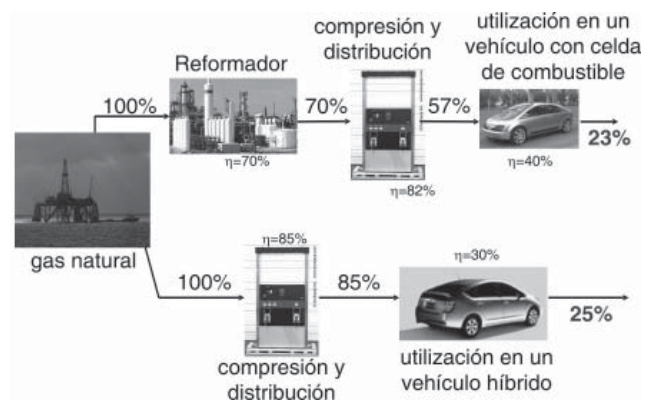
Figura 1. La eficiencia de utilización del gas natural es más alta si se usa directamente en vehículos en vez de convertirse a hidrógeno. Sin embargo, este tipo de análisis de eficiencia total no considera las sinergias que pueden existir en sistemas energéticos.
